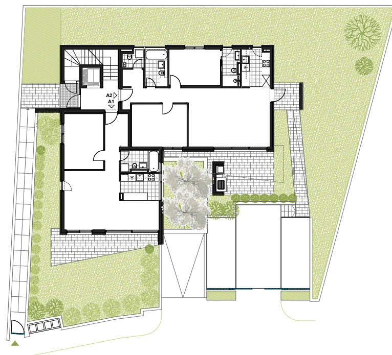
TLOCRT PRIZEMLJA
