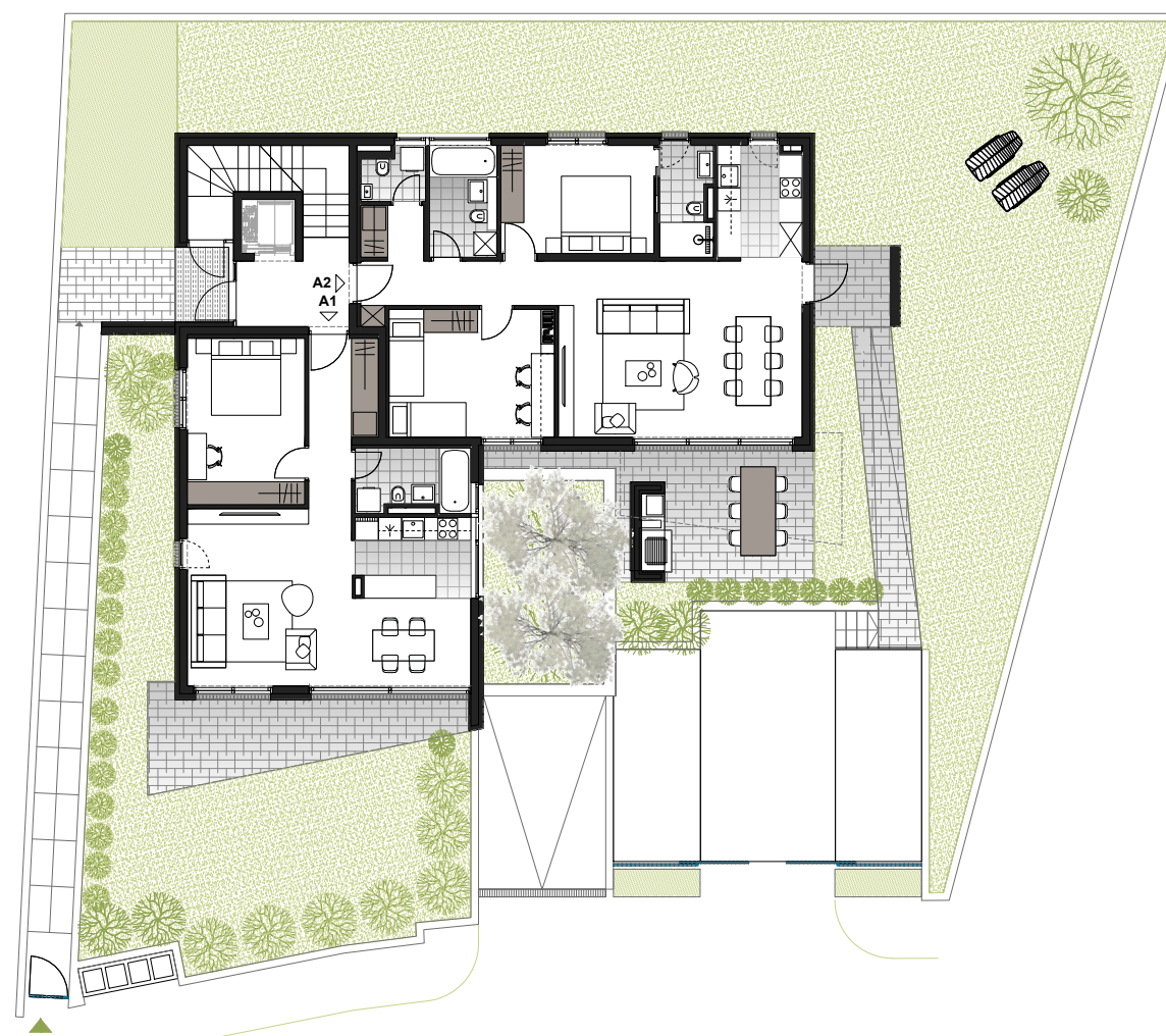
TLOCRT PRIZEMLJA
