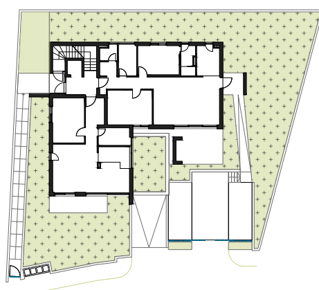
TLOCRT PRIZEMLJA
