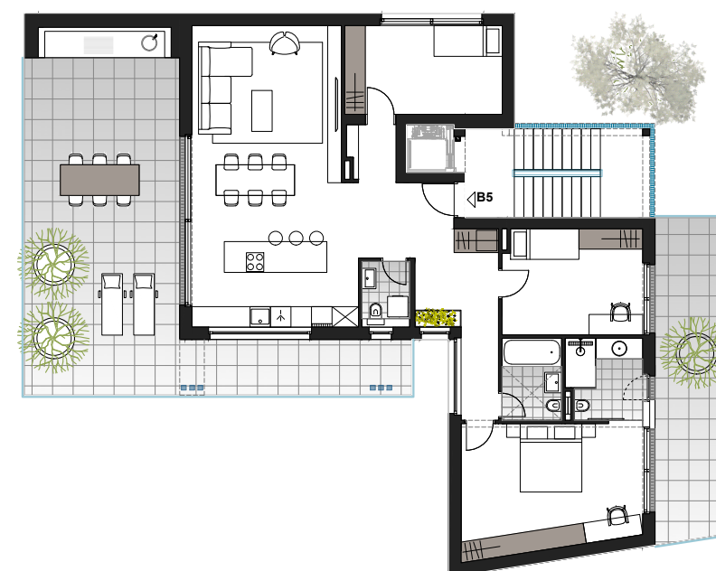
TLOCRT 2. KATA
