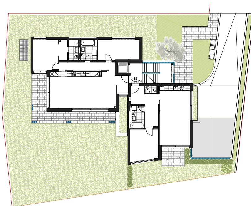
TLOCRT PRIZEMLJA
