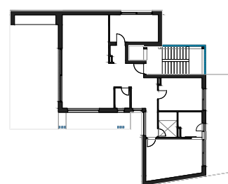
TLOCRT 2. KATA
